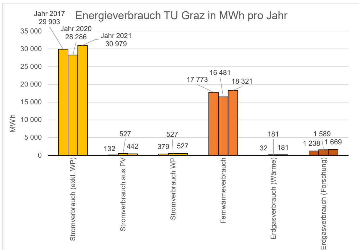
Abbildung 7: Energieverbrauch TU Graz in MWh pro Jahr
