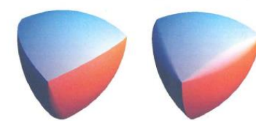
Meissners minimale Gleichdicke auf Basis des Reuleaux-Tetraeders. Die abgerundeten Kanten treffen sich entweder in einem Eckpunkt (unten im linken Bild), oder sie begrenzen eine Fläche (oben im rechten Bild).
